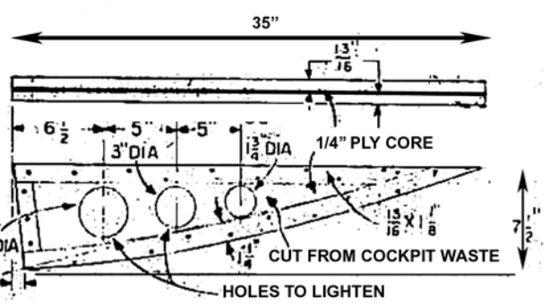
FORE CENTER STRUT 1-REQ
